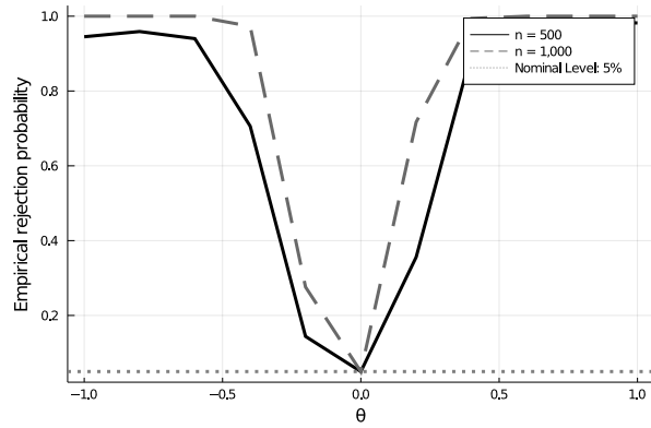
(b) Cramér-von Mises test
