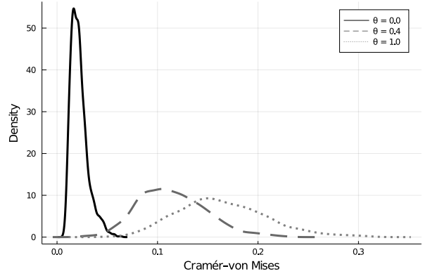
(d) Sample size: n = 1,000
