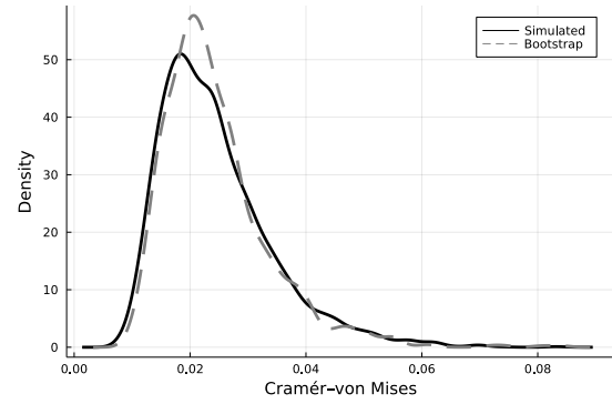
(b) Cramér-von Mises
